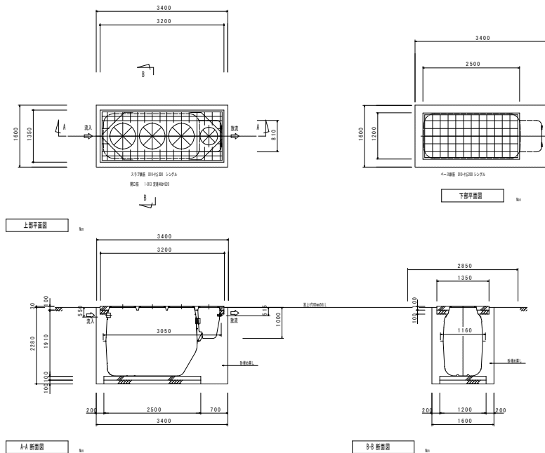
標準施工図 Non
