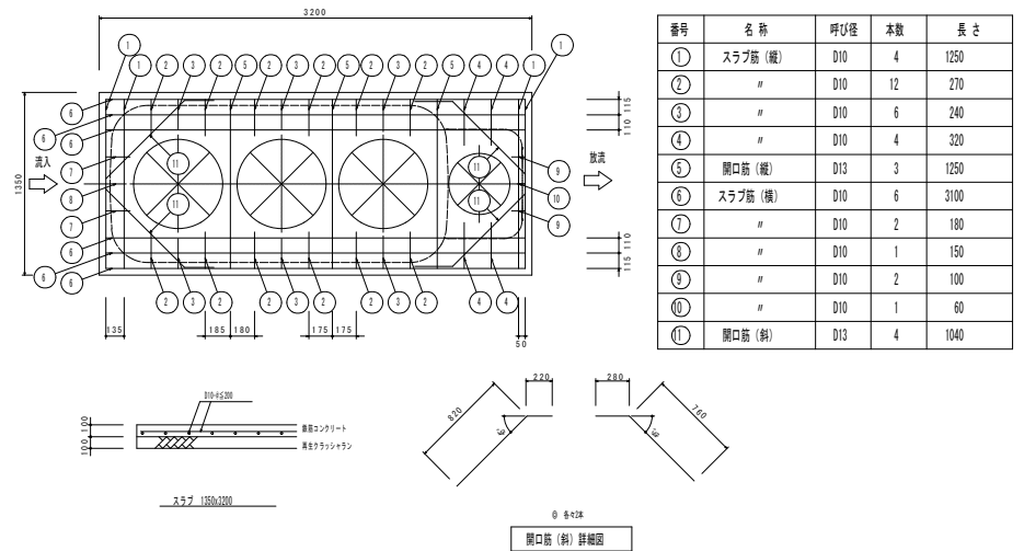
放流管標準施工図 Non
