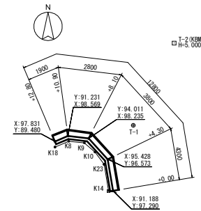
擁壁工配置図
