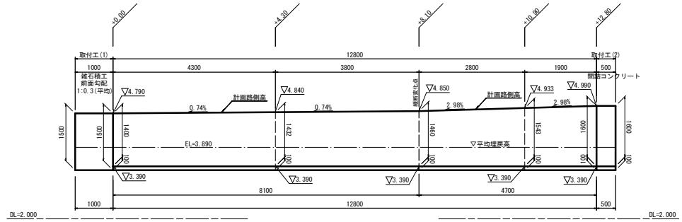
擁壁工展開図
