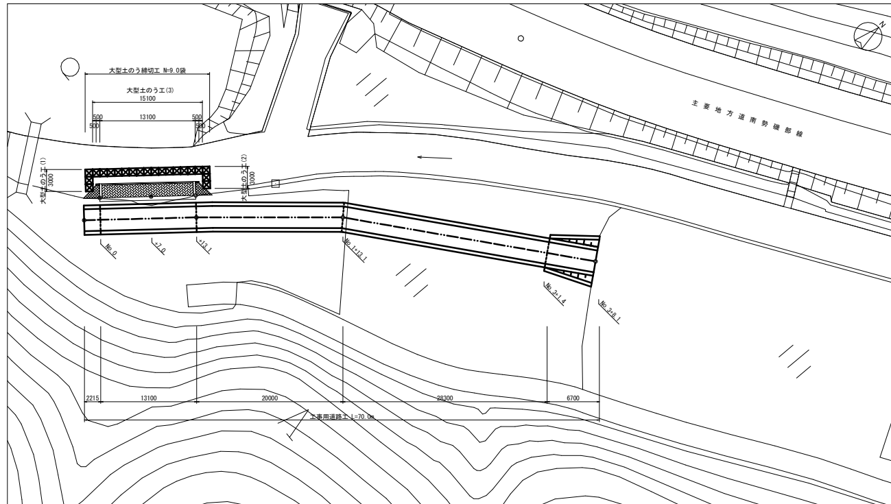
平面图
