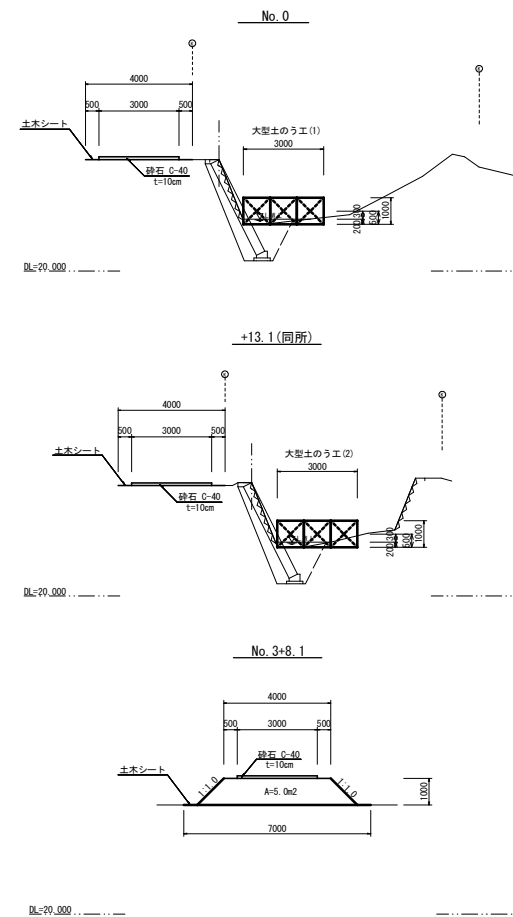
横断面図
