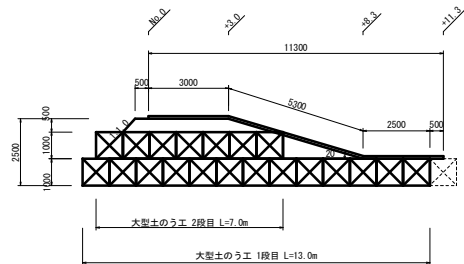
側 面 図 S=1:100
