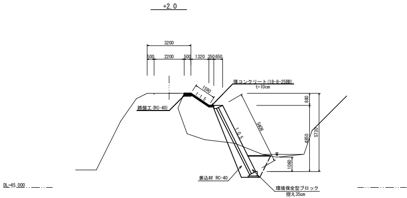
標準断面図 S=1:100
