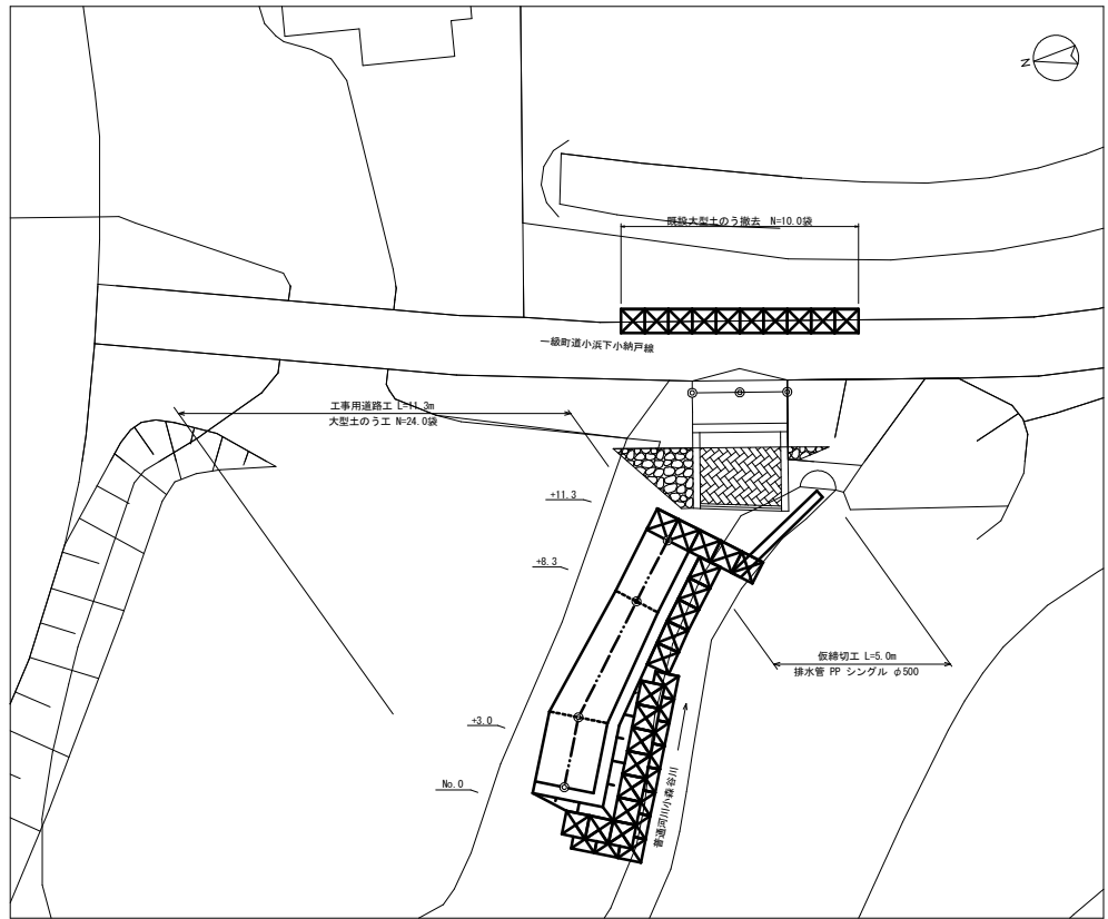
既設大型土のう撤去 S=1:100
