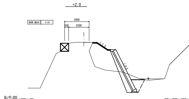
既設大型土のう撤去 S=1:100
