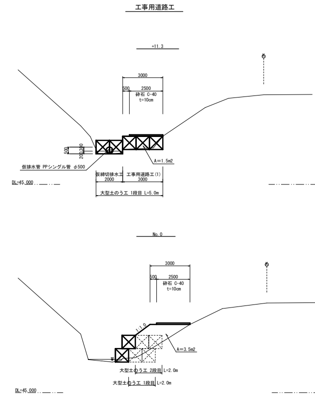
横 断 面 図 S=1:100
