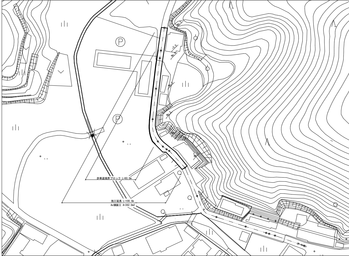
舗装展開図
