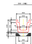
詳細図
