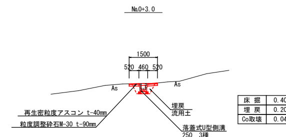
2号箇所標準断面図
