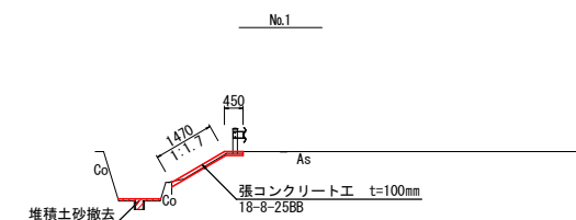
1号箇所標準断面図
