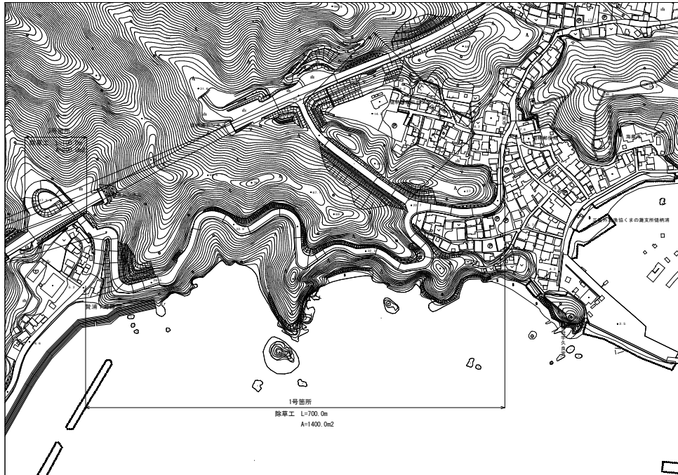
平面図 S=1 : 2500
