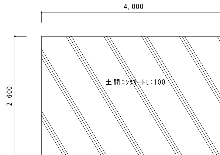
土間伏図 1/50
